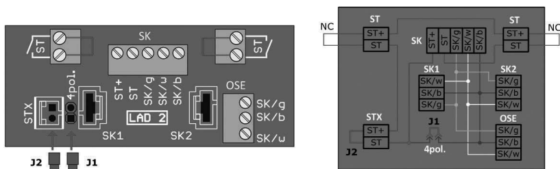
Рисунок 3 – Модуль коммутационный
